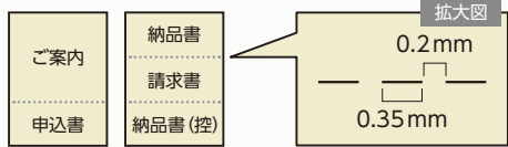
紙折機にセットして使用します。
